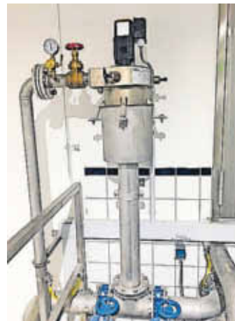
Die Turbine nutzt die Fließgeschwindigkeit des Wassers zur Stromerzeugung.
